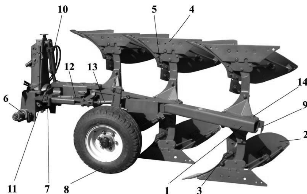
Рисунок 1. Плуг навесной оборотный ПНО-3-40/55
