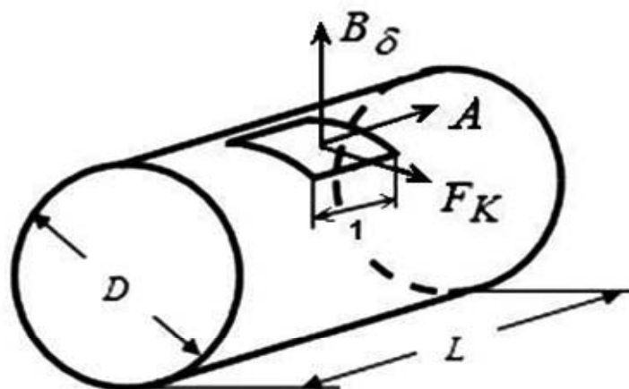
Рисунок 1. Определение средней касательной силы
