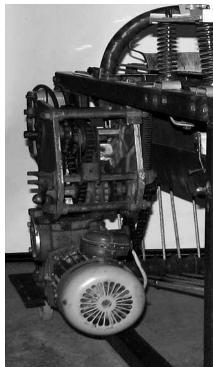
Рисунок 4. Устройство привода
