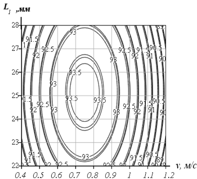
Рисунок 7. График линий уровня общей точности сортирования
