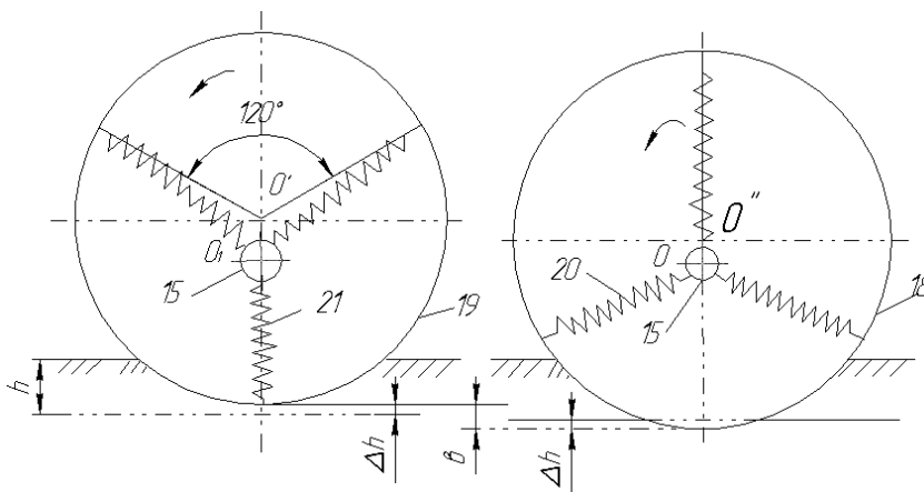
Рисунок 2. Схема относительных вертикальных колебаний соседних заходов спиралей
