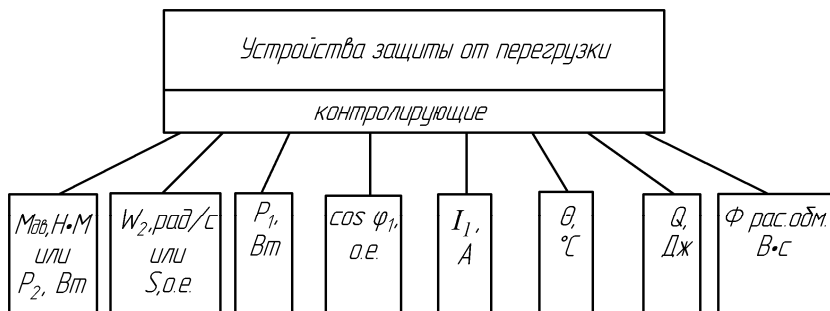
Рисунок 1. Параметры, позволяющие контролировать перегрузку электродвигателя.
